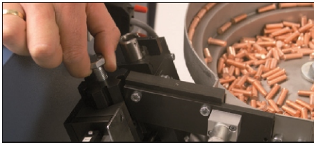
转换其他螺柱直径的快速转换系统 (专利号: DE 199 34 209 C2)
